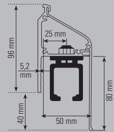
Profilkit 1-spurig
