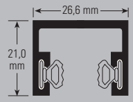
Führungsschiene unten mit Gleitkeder
