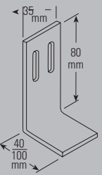
40 / 60 / 100 mm Befestigungswinkel zu Gleiter
