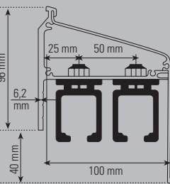
Profilkit 2-spurig
